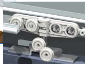
Nosné vozíčky s kuličkovými ložisky nosnost 120 kg
