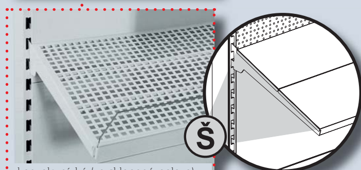
konzola nízká (ve sklopené poloze)
