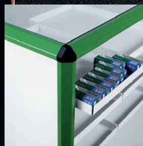
detail rohovníku a spojení profil - plocha (sklo, deska a volný prostor)
