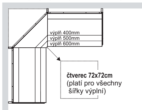
koutový regál (se stojinami 80x30mm)
