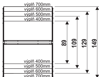
oboustranný regál (se stojinami 60x30mm)
