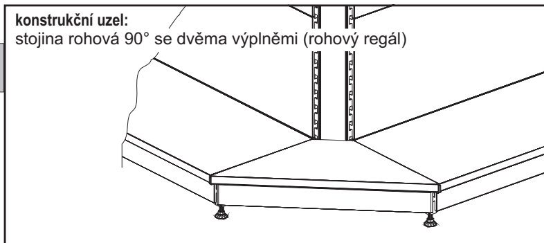
rohový regál (se stojinami 80x30mm)
