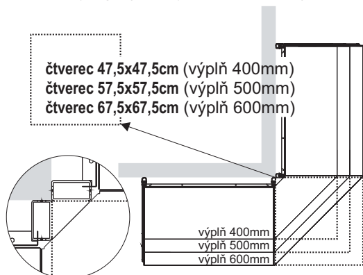
rohový regál (se stojinami 60x30mm)
