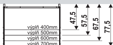
přístěnný regál (se stojinami 60x30mm)
