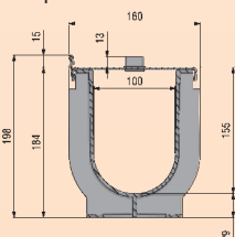
štěrbínový žlab SPORTFIX Super s rozdělovací hranou
