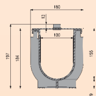
štěrbínový žlab SPORTFIX Super s rozdělovací hranou
