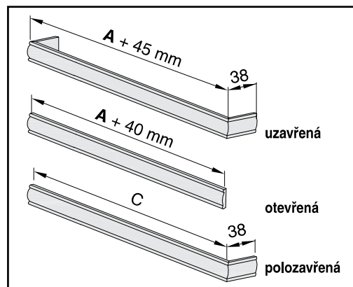
GARNÝŽ - BOČNICE
