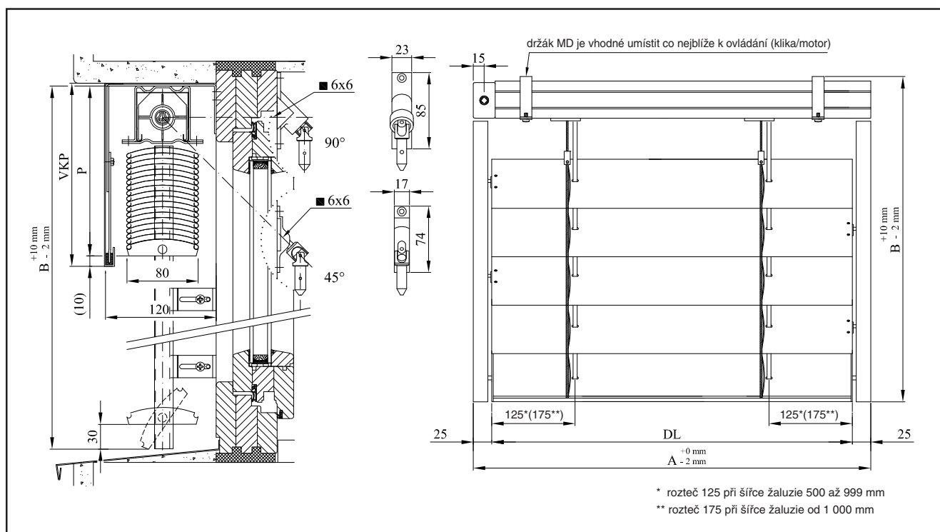
C-80 - Vedení v lištách
