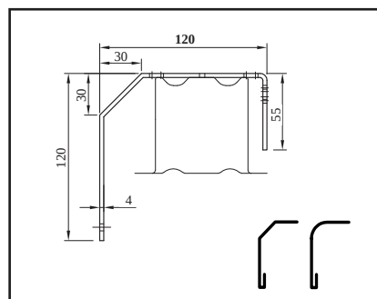
DK 3a - Držák krycího plechu zkosený pro C-80, Z-70, F-80
