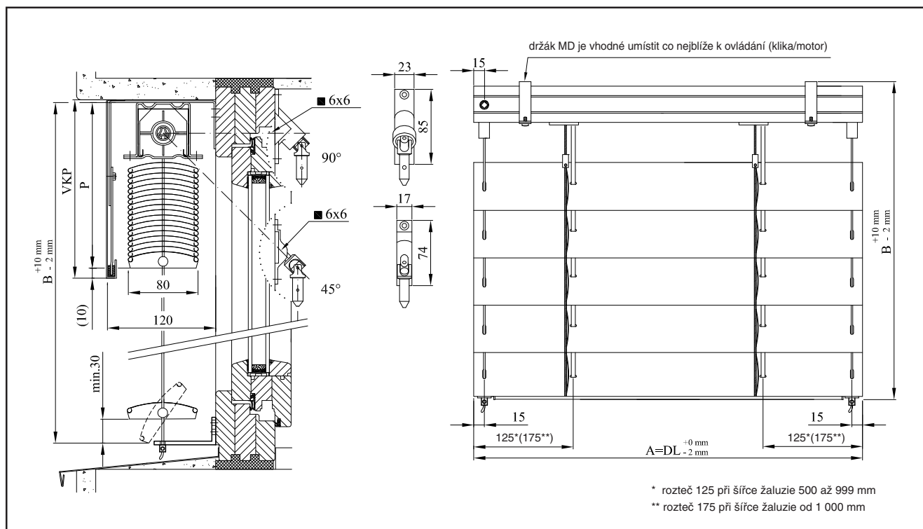
C-80 - Vedení v lanku
