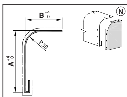
KP 1e L = A + B
