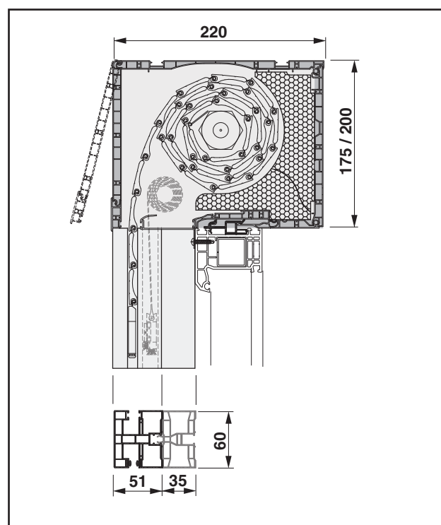
Vnější revizní klapka (box 175 / 200 X 220)
