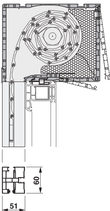
Standardní provedení (vnitřní / spodní - revizní klapka)
