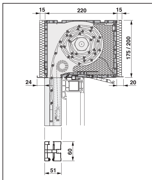
Oboustranné podomítkové provedení, spodní revizní klapka (box 175 / 200 X 220)
