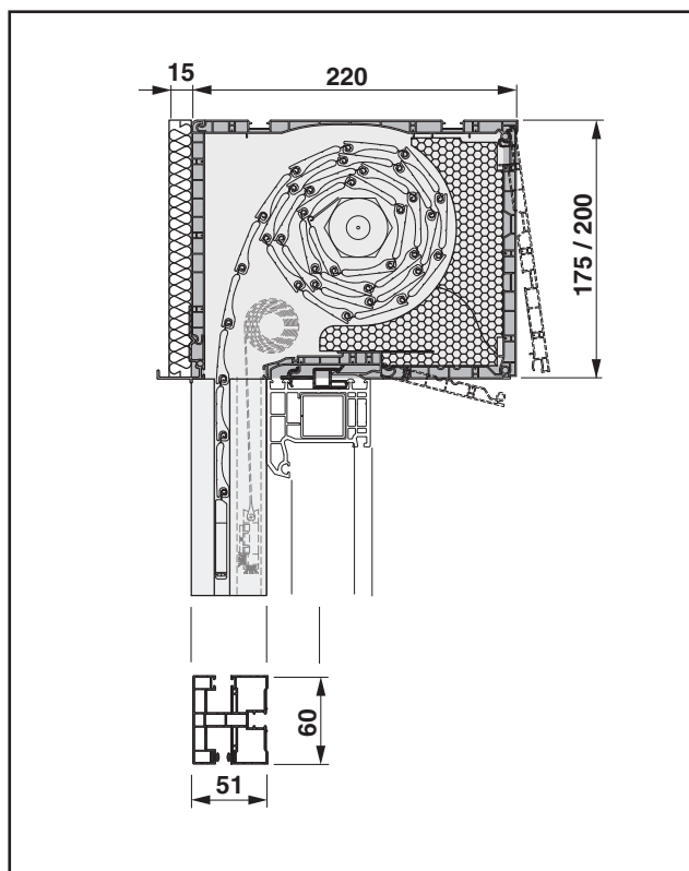
Vnější podomítkové provedení, spodní / vnitřní - revizní klapka (box 175 / 200 X 220)
