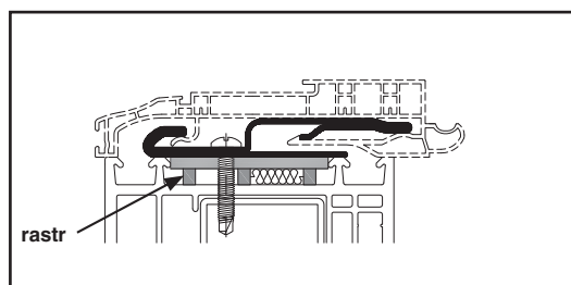
Adaptér kovový s rastrem - PVC okna
