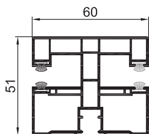
Vodící lišta PVC
