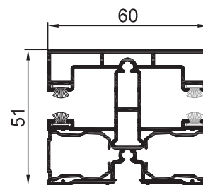
Vodící lišta Al
