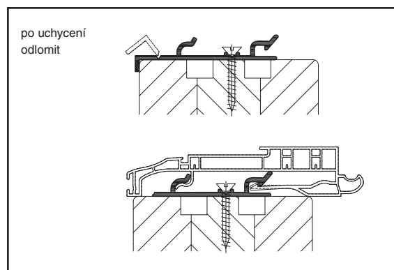
Adaptér PVC univerzal - Euro okna
