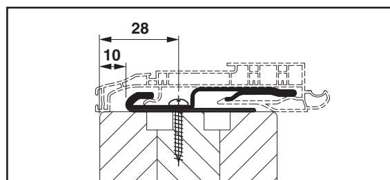
Adaptér kovový - Euro okna
