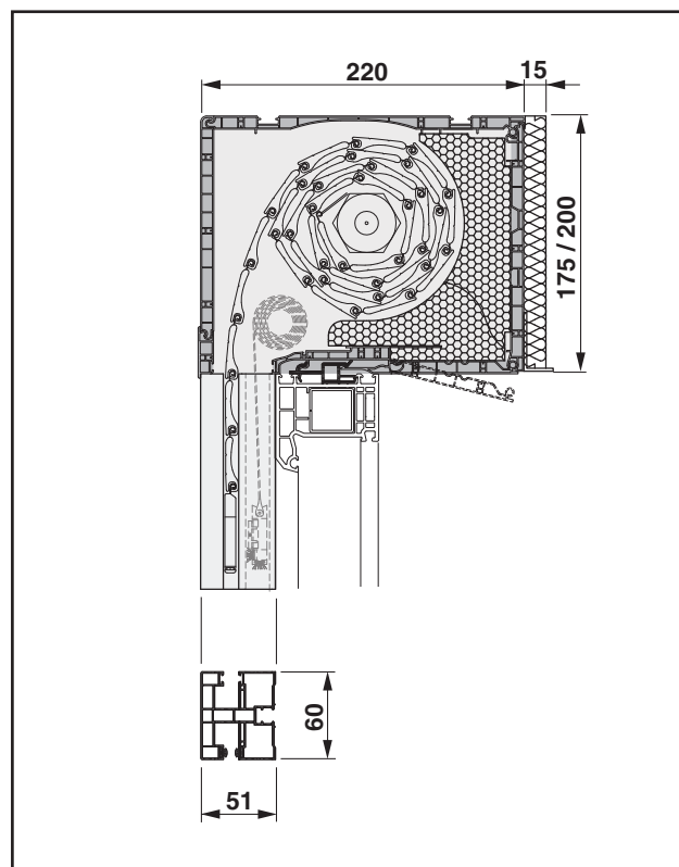
Vnitřní podomítkové provedení, spodní - revizní klapka (box 175 / 200 X 220)
