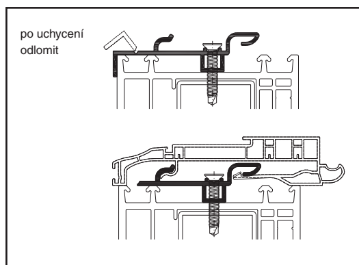
Adaptér PVC univerzal - PVC okna
