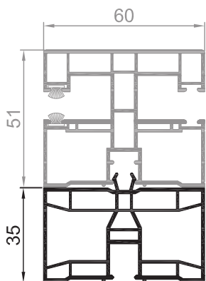
Odsazovací PVC profil
