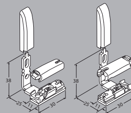
Úhelník na zasklívací lištu VS, pár 48210 šedá 48211 bílá 48212 černá VS 1 a VS 3 = max. šířka plisé 50 cm
