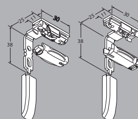
Držák rohový a botička se zajištěním, pár 49210 šedá 49211 bílá 49212 černá VS 1, VS 3 a VS 3 SD = max. šířka plisé 50 cm
