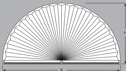
SR 1: Šířka, výška (radius = 1/2 šířky)
