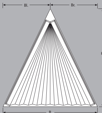
SDP 3: Šířka, výška, šikmina vlevo, šikmina vpravo
