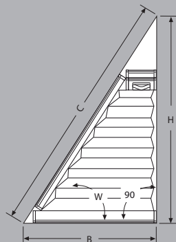
PL 33, PL 33 D, PLK 33, PLE 33 (obr. PL 33)
