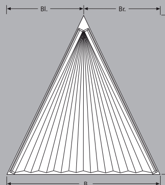
SD 3: Šířka, výška, šikmina vlevo, šikmina vpravo
