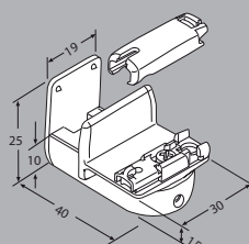
Upínací držák s botičkou 48333 šedá 48334 bílá 48335 černá Příplatek: 117 Kč / ks
