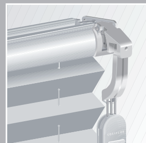
Brzda a zarážka pro F - plisé
