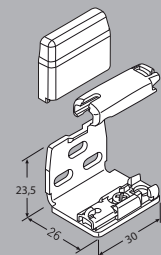
Úhelník s botičkou 48224 šedá 48225 bílá 48226 černá
