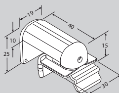
Upínací držák 48300 šedá 48301 bílá 48302 černá Příplatek: 117 Kč / ks
