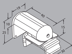
Upínací držák 48300 šedá 48301 bílá 48302 černá Příplatek: 117 Kč / ks
