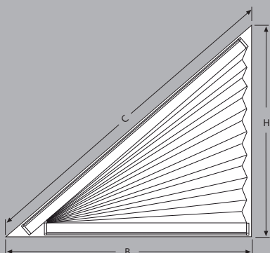
SDP 2: Šířka, výška, šikmina
