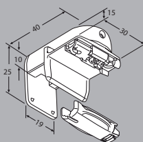
Upínací držák s botičkou se zajištěním 49333 šedá 49334 bílá 49335 černá Příplatek: 117 Kč / ks
