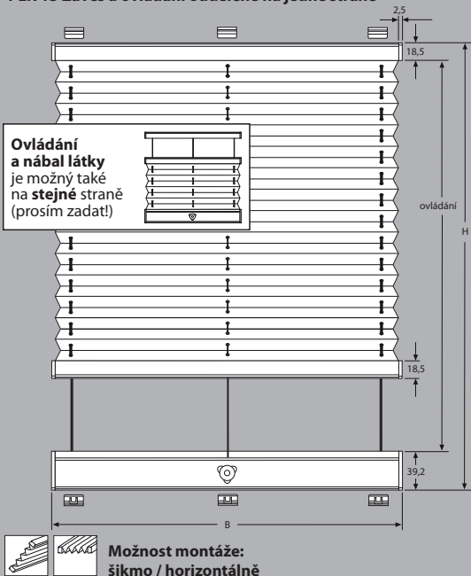
PLK 13 Závěs a ovládání oddělené na jedné straně
