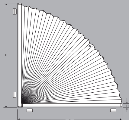
SR 2 - fixní šířka = radius
