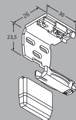
Úhelník a botička se zajištěním 49124 šedá 49125 bílá 49126 černá
