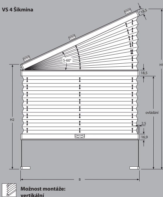
VS 4 Šikmina S Plně ovladatelná
