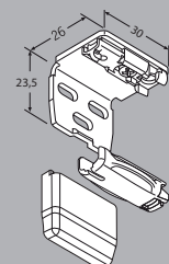
Úhelník a botička se zajištěním 49224 šedá 49225 bílá 49226 černá
