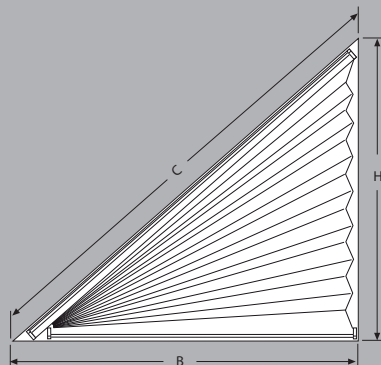
SD 2: Šířka, výška, šikmina
