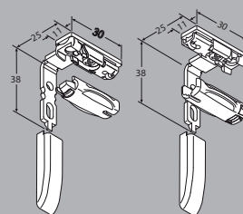
Úhelník na zasklívací lištu VS 1 a VS 3, pár 48213 šedá 48214 bílá 48215 černá VS 1 a VS 3 = max. šířka plisé 50 cm
