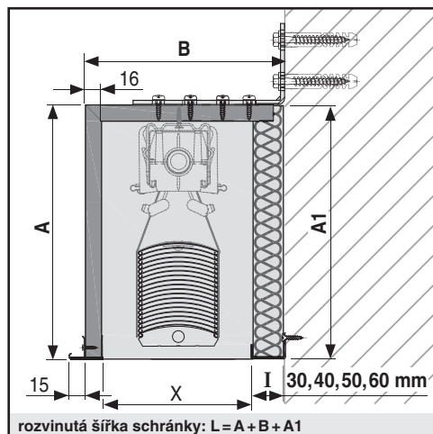
PSI - s izolací 30, 40, 50, 60 mm
