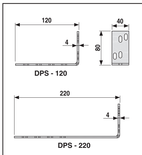
DPS - držák podomítkové schránky
