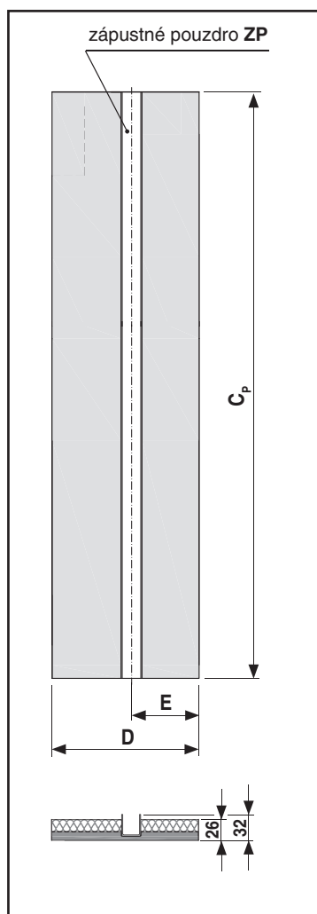
IP 26 - izolační panel 26 mm
