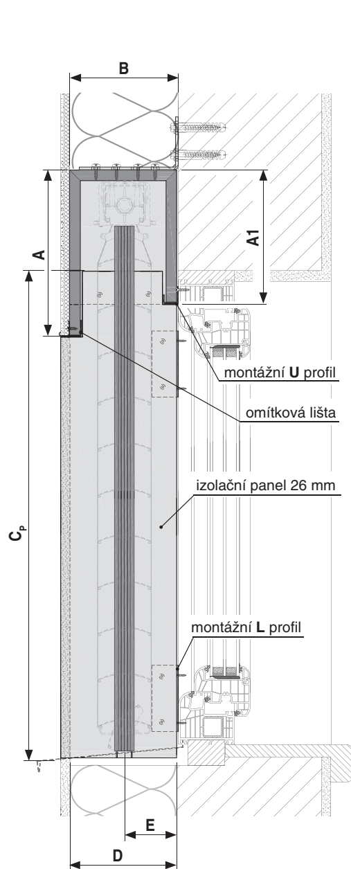
PS - Podomítková schránka (předokenní montáž)
