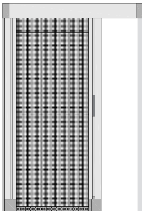
Pohled z montážní strany (bez L profilu)
