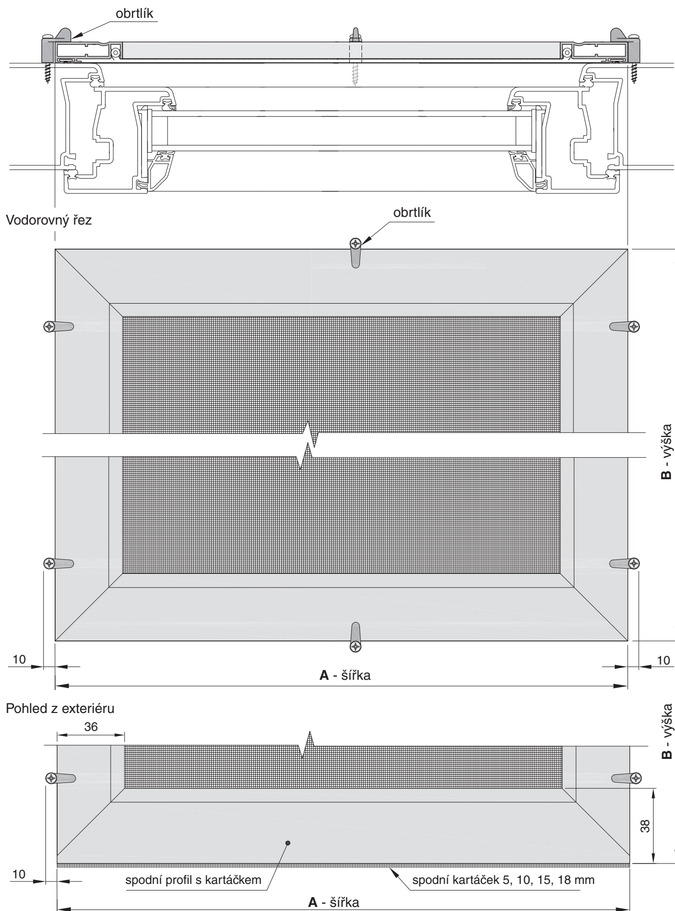
Pohled z exteriéru - provedení spodní kartáček
