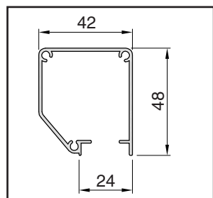
Řez profilem boxu
