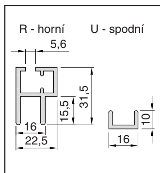
Řezy lišty R, U
