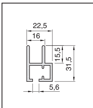
Řez lišty R
