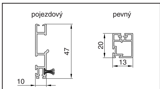
Řezy spodních profilů
