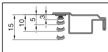
Možnost samolepícího těsnícího kartáčku (příbaleno)
