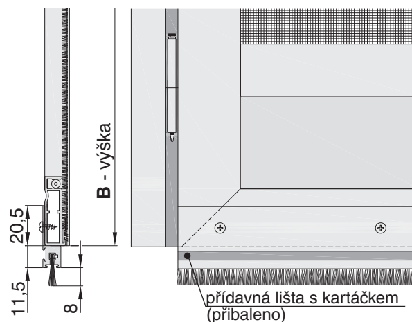
Pohled z montážní strany - provedení: bez spodní části rámu - přídavná lišta s kartáčkem
