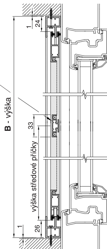
Svislý řez
