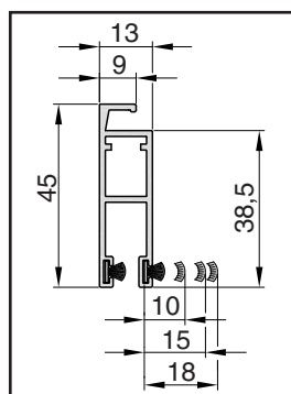
Řez profilem křídla sítě
