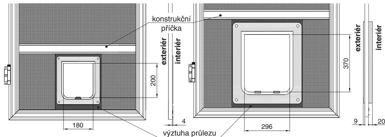
Průlez pro kočku (světlost otvoru 18 x 20 cm)
