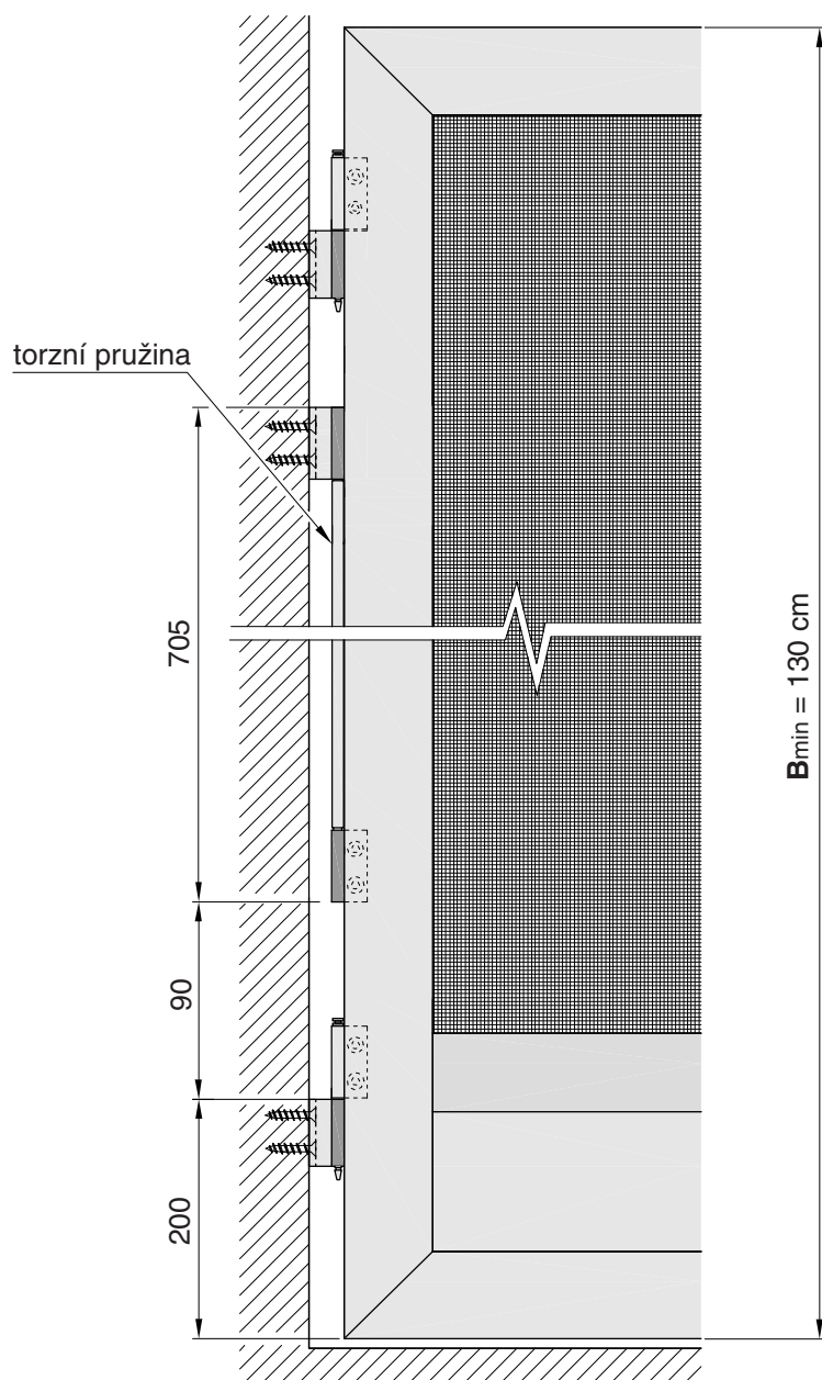
Pohled z boku (otevřené dveře) - samozavírací systém
