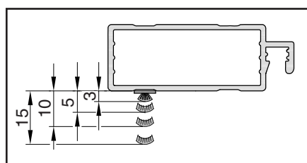
Možnost samolepícího těsnícího kartáčku (příbaleno)
