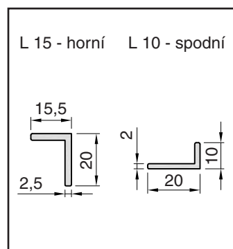
Řezy lišt L 15, L 10
