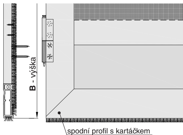
Pohled z montážní strany - provedení: spodní kartáček
