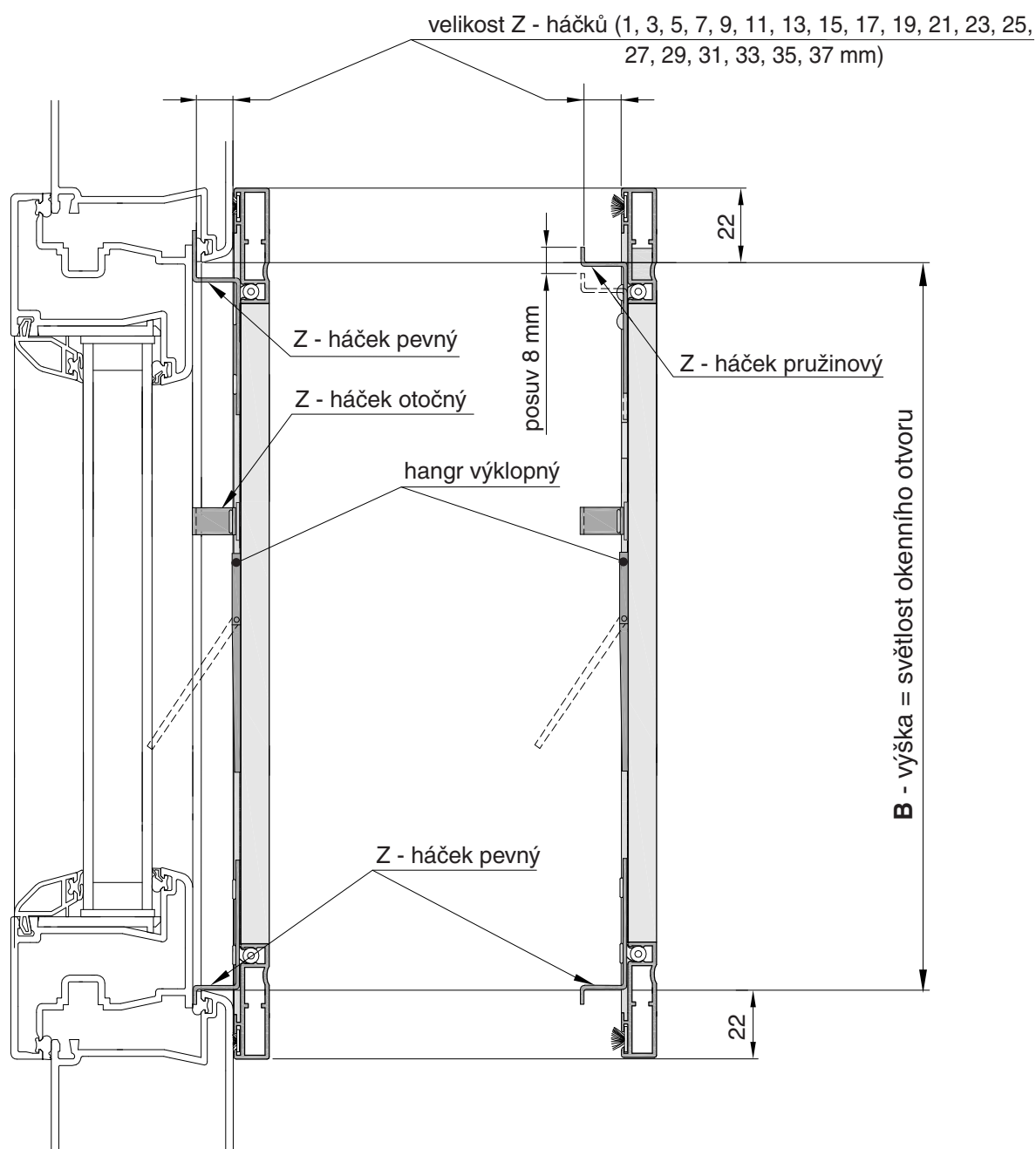
Svislý řez Z - háčky pevné
