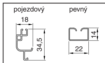
Řezy spodních profilů
