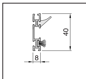
Řez pojezdového profilu
