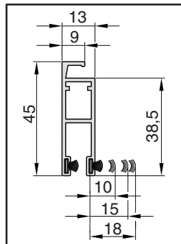
Řez profilem křídla sítě
