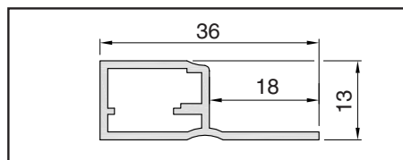
Řez rámovým profilem 36 x 13 mm ULTRA
