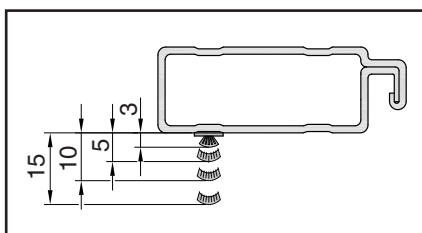
Možnost samolepícího těsnícího kartáčku (přibaleno)
