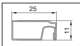
Řez profilem 25 mm
