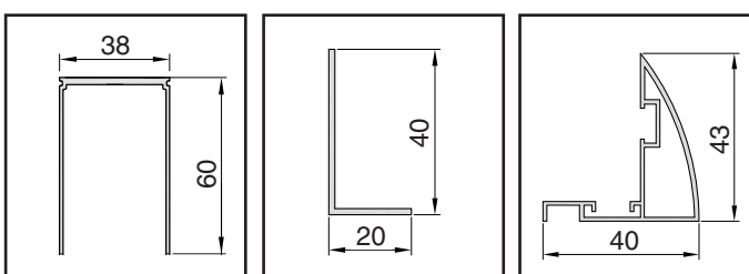
Řez horním profilem
