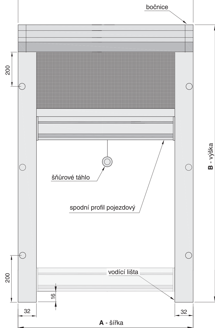
Pohled z montážní strany
