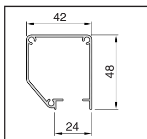
Řez profilem boxu
