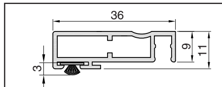
Řez profilem 36 x 11 mm ULTRA
