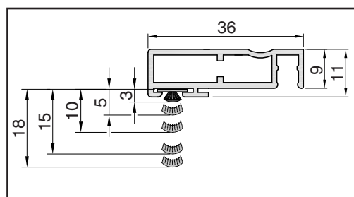
Řez profilem 36 mm
