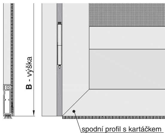
Pohled z montážní strany - provedení: bez spodní části rámu - spodní kartáček
