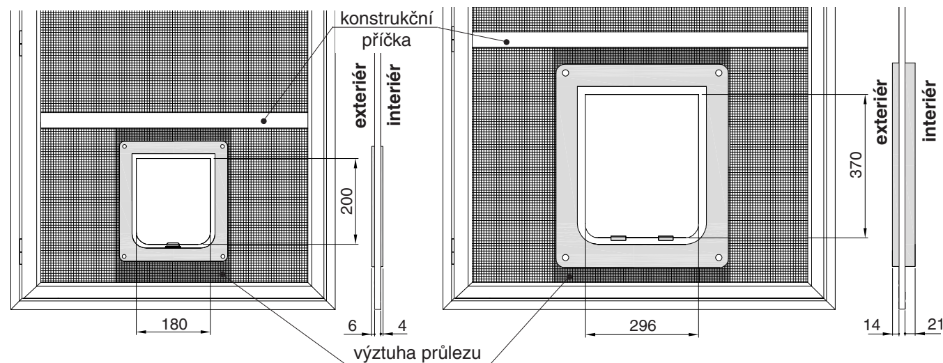
Průlez pro kočku (světlost otvoru 18 x 20 cm)
