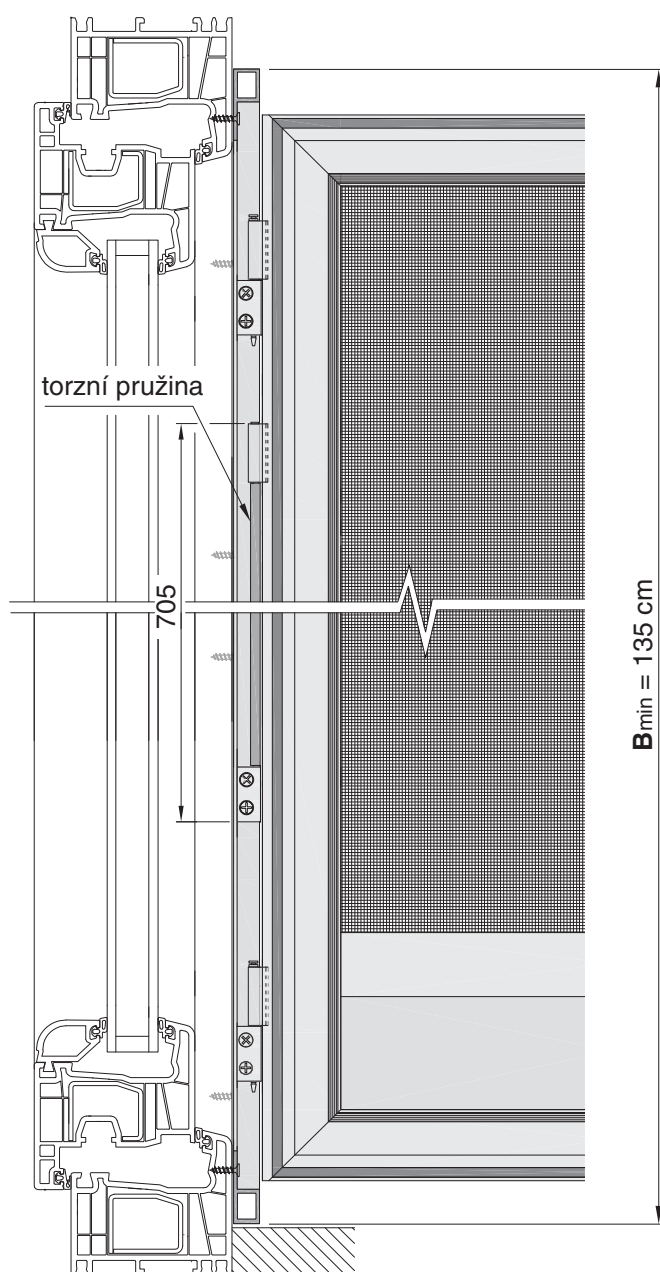
Pohled z boku (otevřené dveře) - samozavírací systém
