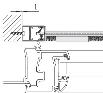
Vodorovný řez - montáž do ostění
