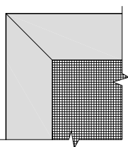
Pohled z exteriéru (vnitřní roh)
