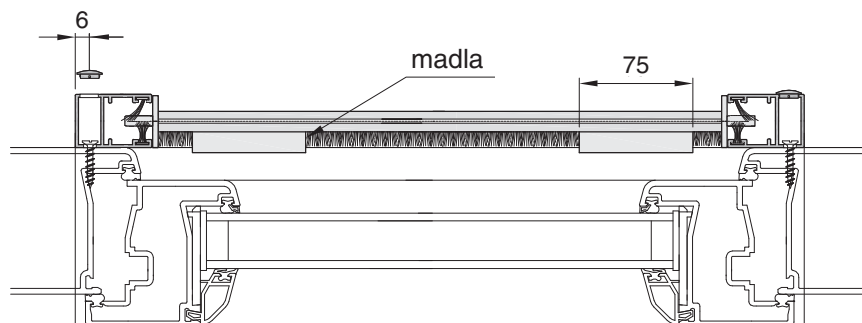
Vodorovný řez - montáž na rám
