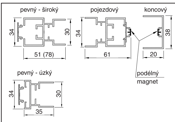
Řezy svislými profilem
