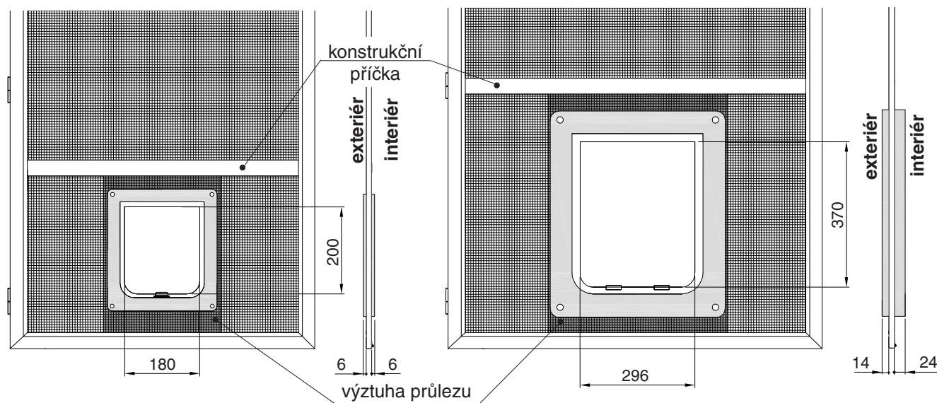
Průlez pro kočku (světlost otvoru 18 x 20 cm)
