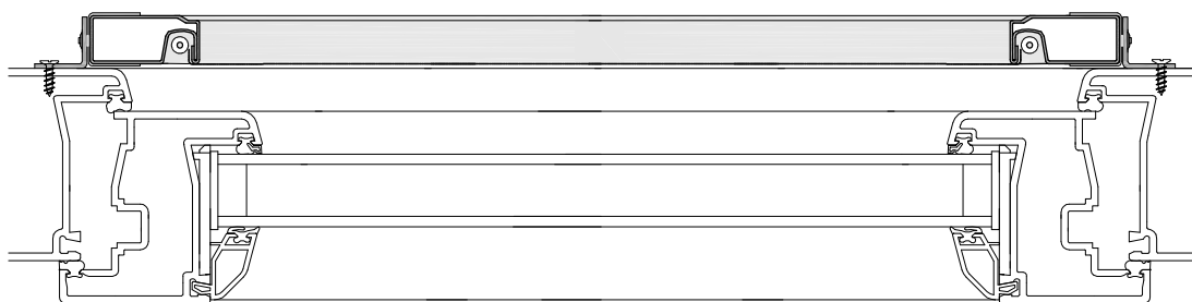
Vodorovný řez
