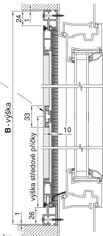
Svislý řez
