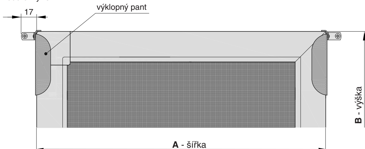
Pohled z exteriéru
