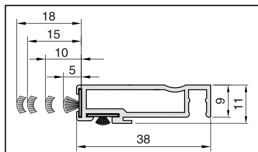
Možnost profilu s těsnícím kartáčkem
