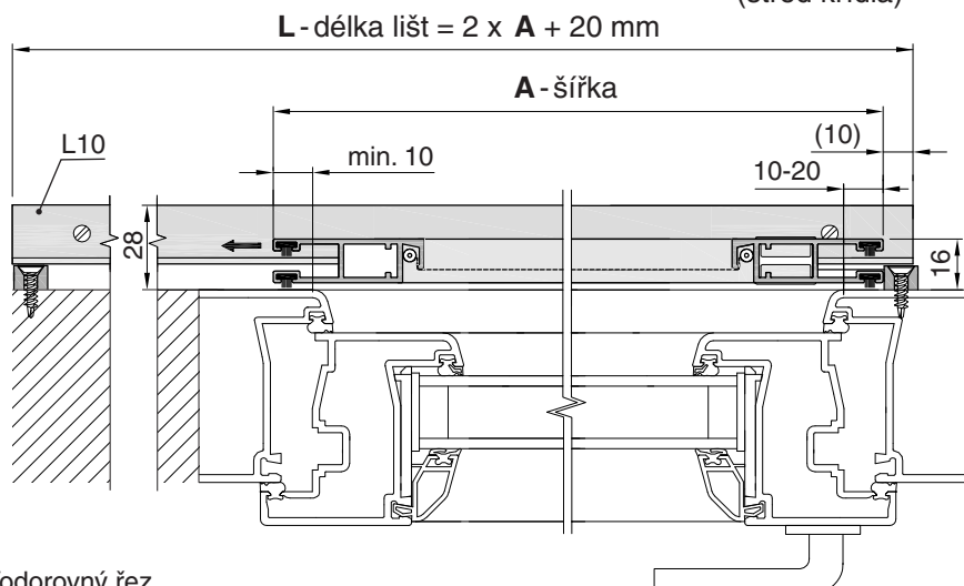
Vodorovný řez
