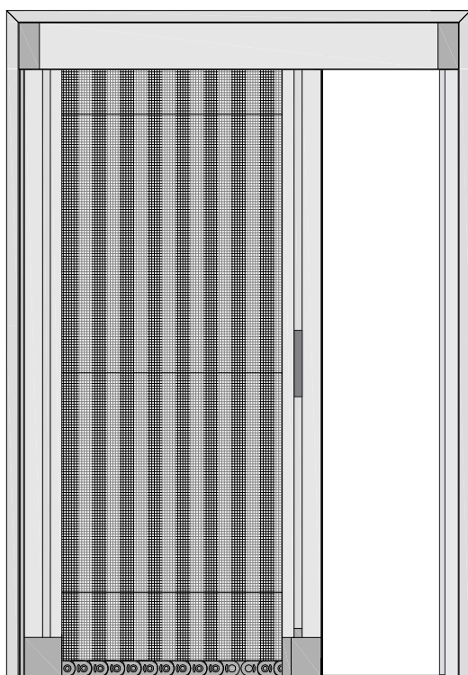
Pohled z montážní strany (provedení s L profilem)
