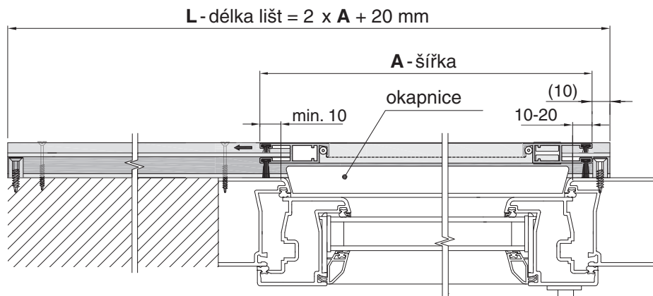
Vodorovný řez
