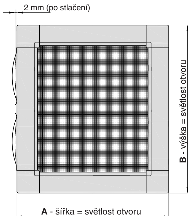
Pohled z exteriéru - vnější roh
