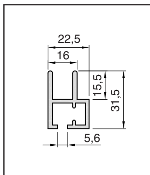
Řez rámu R
