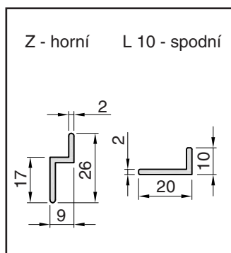
Řezy lišt Z, L
