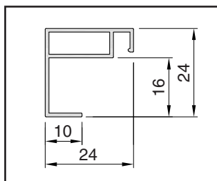
Řez profilem odsazeným
