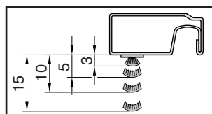
Možnost samolepícího těsnícího kartáčku (příbaleno)
