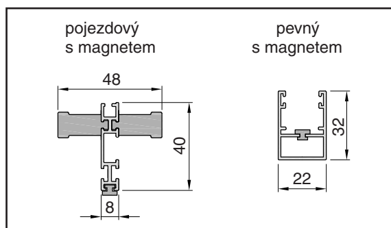
Řezy profilů
