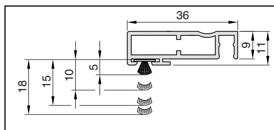
Řez profilem 36 x 11 mm EXTRA
