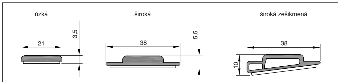
Spodní samolepící PVC kolejnice
