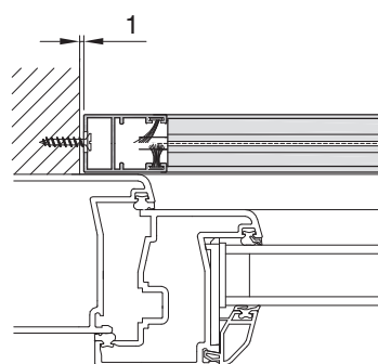
Vodorovný řez - montáž do ostění
