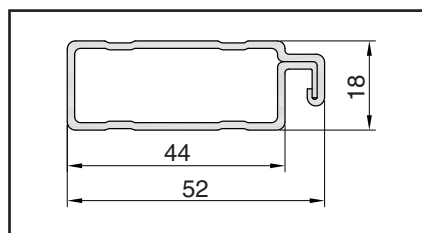
Řez profilem 52 x 18 mm
