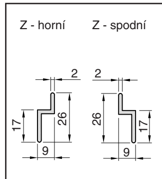
Řezy lišt Z, Z
