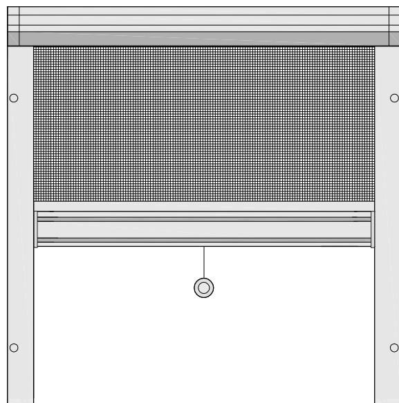
Pohled z montážní strany
