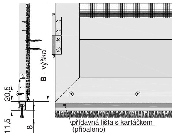
Pohled z montážní strany - provedení: přídavná lišta s kartáčkem
