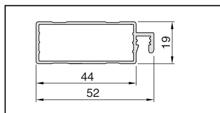
Řez profilem 52 x 19 mm
