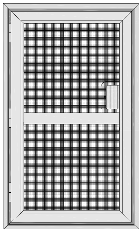
Pohled z montážní strany
