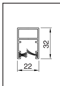
Řez vodící lišty
