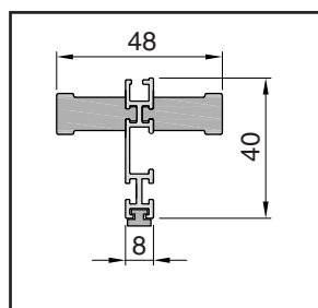
Řez pojezdového profilu s magnetem
