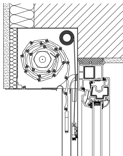
Podomítkový box 90° – roleta kombinovaná se sítí
