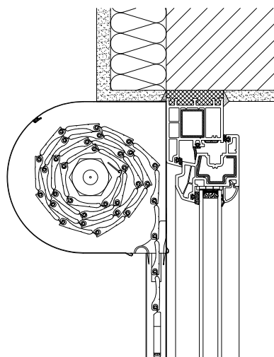
Předokenní roleta – kulatý box
