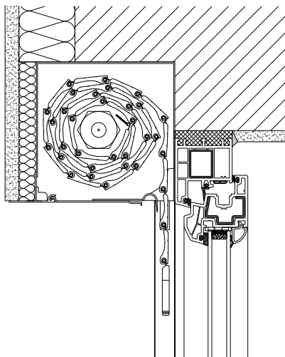
Podomítkový box 90°
