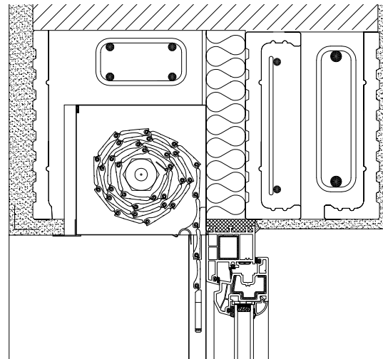
Roleta v překladu RONO
