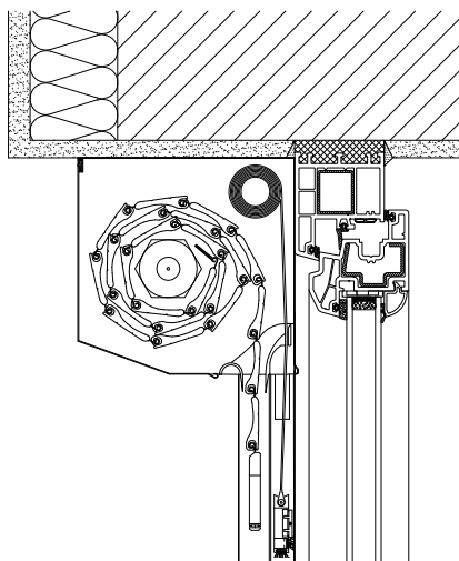
Předokenní roleta kombinovaná se sítí – box 20°
