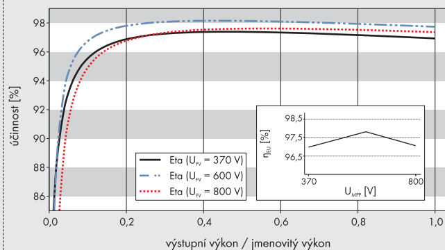
Křivka účinnosti SUNNY TRIPOWER 9000TL
