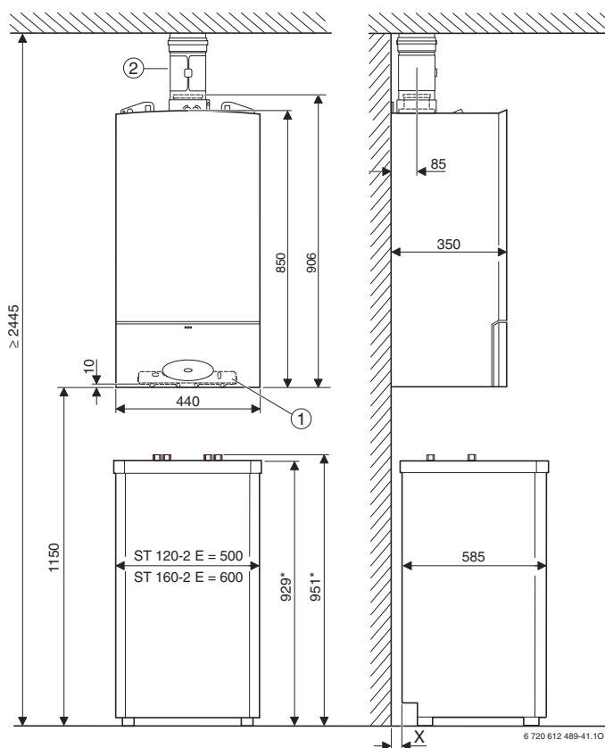
Rozměrový výkres CerapurComfort
