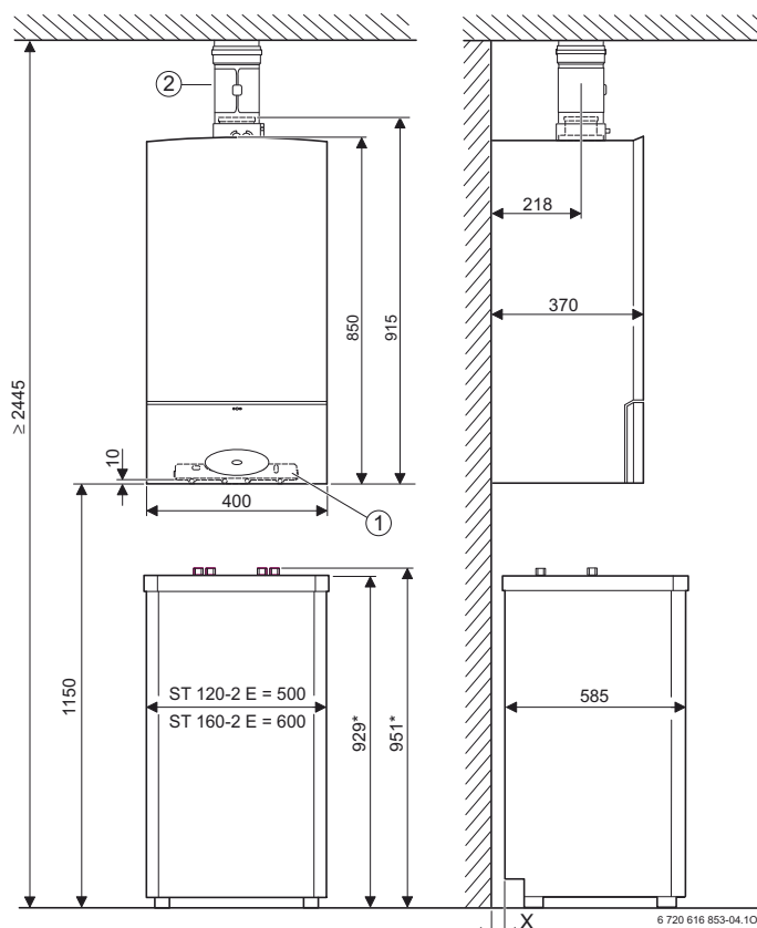
Rozměrový výkres CerapurSmart
