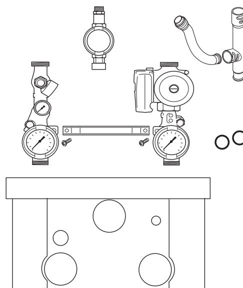
Čerpadlová skupina
