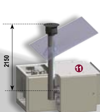
Odtah pouze spalin B22 max. délka : 8 m
