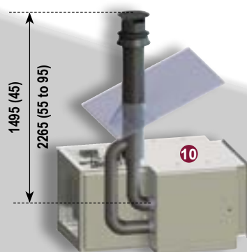
Koncentrický otať přes strop C32 max. délka : 8 m
