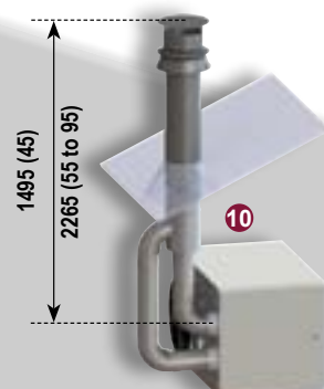
Koncentrický odtah přes strop C32 max. délka : 8 m
