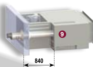
Koncentrický otať přes zeď C12 max. délka : 6 m
