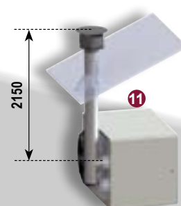
Odtah pouze spalin B22 max. délka : 8 m
