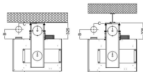
Montáž na zeď
