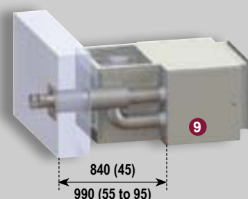
Koncentrický otať přes zeď C12 max. délka : 6 m
