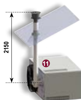
Odtah pouze spalin B22 max. délka : 8 m
