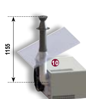
Koncentrický odtah přes strop C32 max. délka : 6 m
