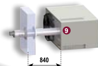
Koncentrický odtah přes zeď C12 max. délka : 6 m
