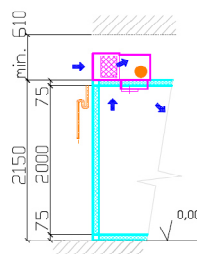
ŘEZ MINI-R (P)
