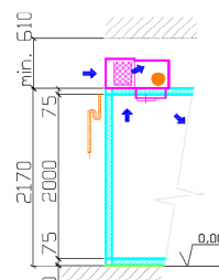
ŘEZ MINI-R (N)
