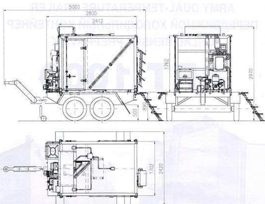
Basic dimensions in mm / Габаритные размеры в мм / Základní rozměry v mm
