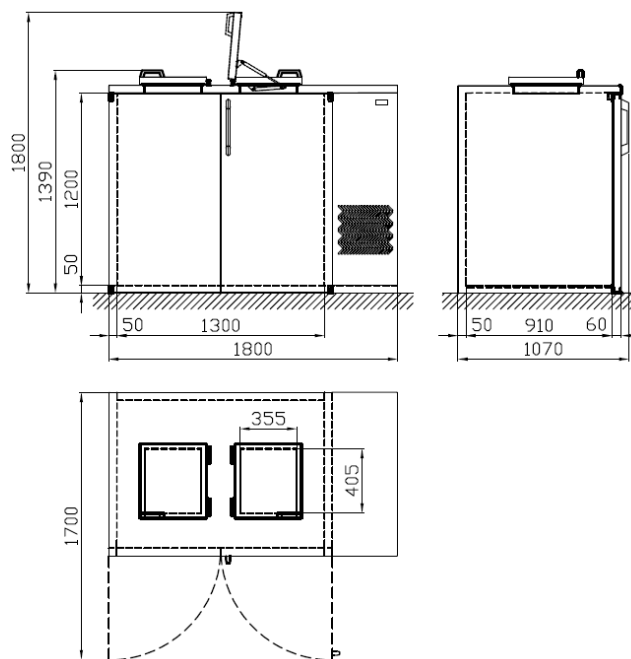
Chladicí skříň CHS-O2
