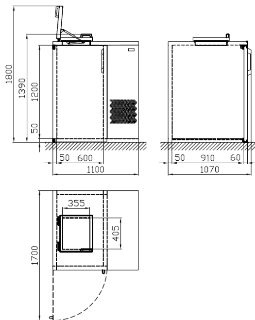
Chladicí skříň CHS-O1
