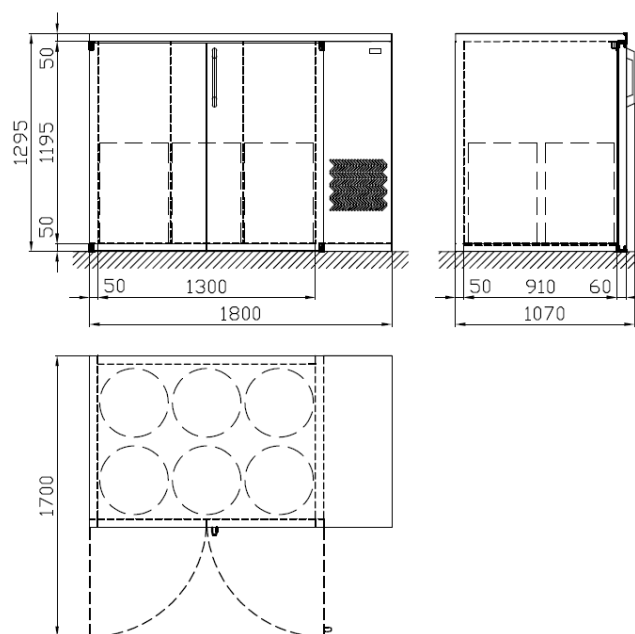
Chladicí skříň CHS-P2
