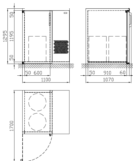
Chladicí skříň CHS-P1
