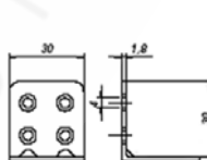
Úhelník nábytkový UP5 / Corner plate UP5
