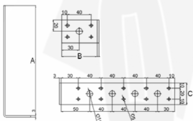
Úhelník kotevní UK2 / Anchoring plate UK2
