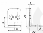
Úhelník nábytkový UN2 / Cabinet support UN2
