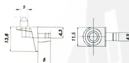
Podpěra policová P4 / Shelf support P4
