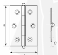
Závěs lomený s volným čepem / Bent hinge with loose pin
