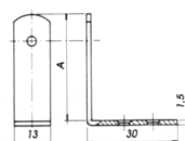
Úhelník nábytkový UN1 / Cabinet support UN1
