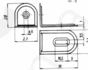
Úhelník nábytkový UN3 / Cabinet support UN3
