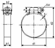
Spona hadicová W1 / Hose clamp W1
