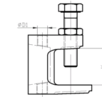
Závěs na nosník / Beam support
