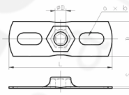
Deska patní / Base plate
