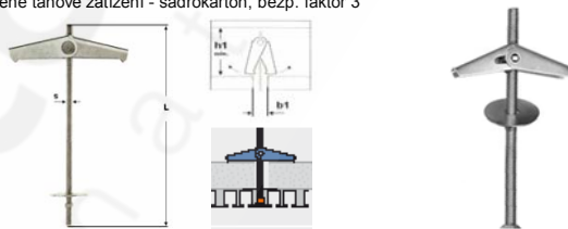
Kotva rozpěrná se šroubem / Spring toggle with bolt
