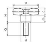
Kolečko se šroubem (stavitelná nožička) / Wheel with bolt
