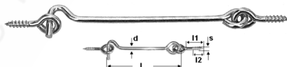
Hák rozpěrný s okem / Gate hook
