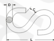
S hák s oplastovanými konci / S hook with end-covers
