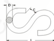
S hák s oplastovanými konci otočený o 90° / Twisted S hook with end-covers
