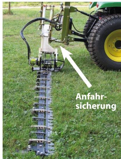
mechanische Anfahr-sicherung
