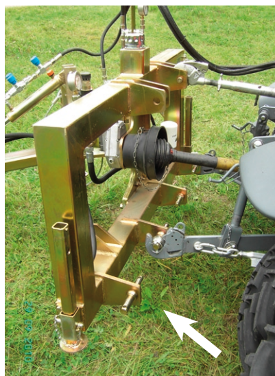
Koppel-Dreipunkt seitenversetzt
