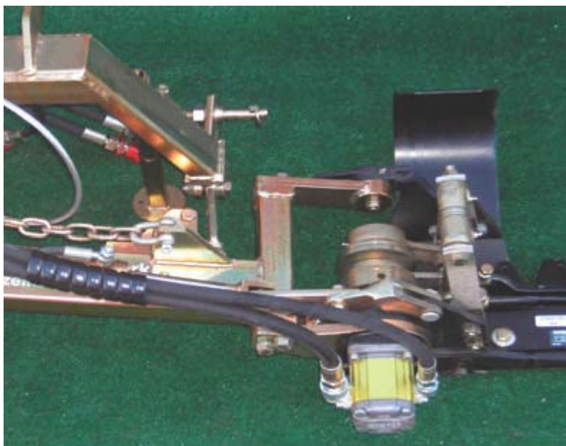
DMH-H- 1,65 m hydraulický pohon kosy. Hydromotor je poháněn přes hydraulický systém traktoru.
