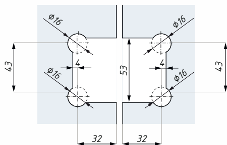
Příprava skla Glass preparation
