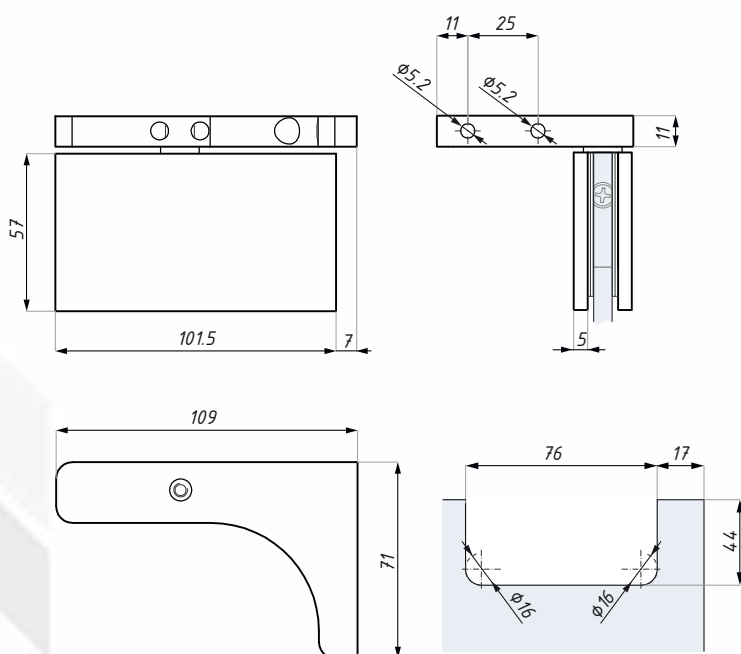
Příprava skla Glass preparation
