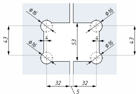
Příprava skla Glass preparation
