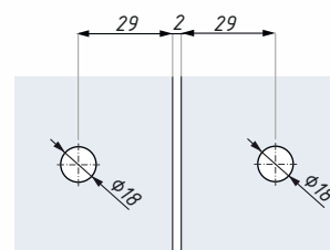
Příprava skla pro nastavení 180 ° Glass preparation for 180 °
