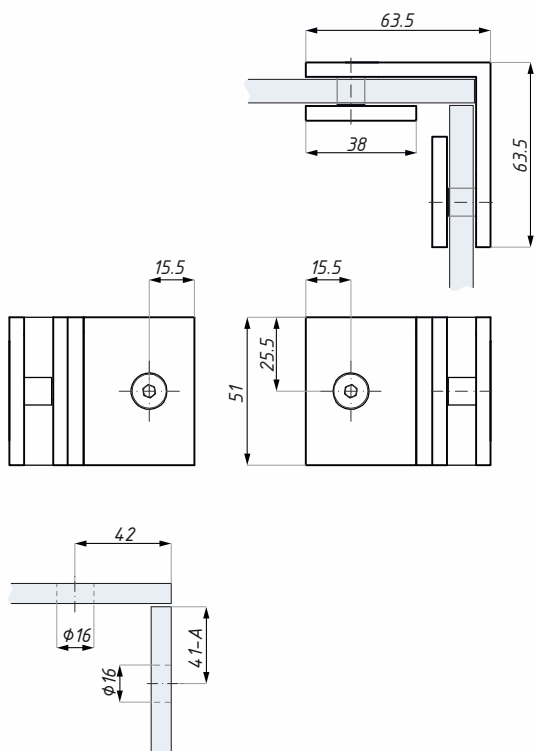
Příprava skla Glass preparation
