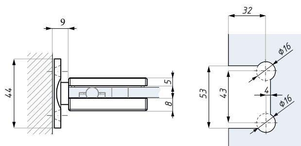
Příprava skla Glass preparation
