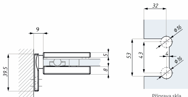
Příprava skla Glass preparation
