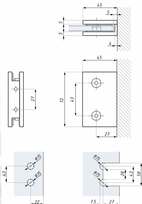
Příprava skla pro mezeru 5 mm Glass preparation: gap 5 mm
