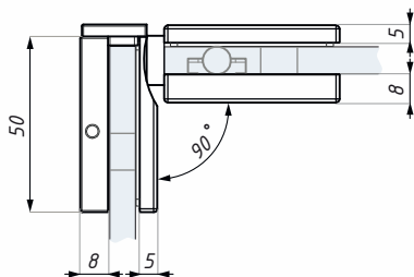
Příprava skla Glass preparation
