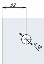
Příprava skla pro nastavení 90° Glass preparation for 90°
