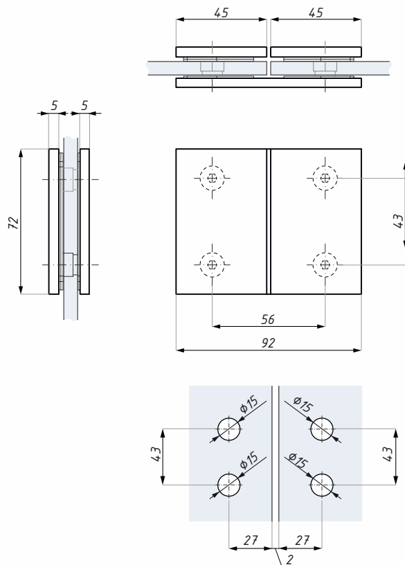
Příprava skla Glass preparation
