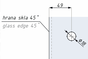
Příprava skla pro nastavení 45° Glass preparation for 45°
