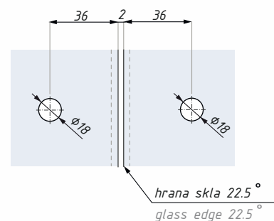
Příprava skla pro nastavení 135 ° Glass preparation for 135 °
