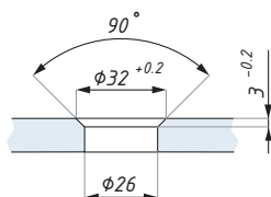
Příprava skla pod bodový úchyt zapuštěný Glass preparation for countersunk routel
