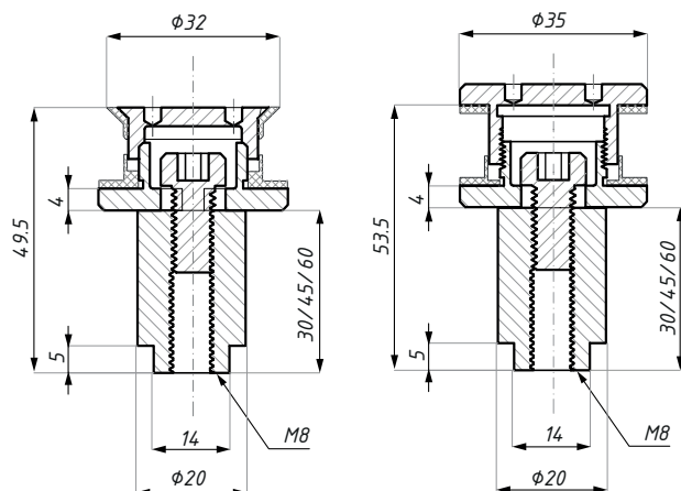
úchyt zapuštěný CSA CSA countersunk routel
