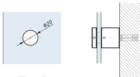
Příprava skla Glass preparation
