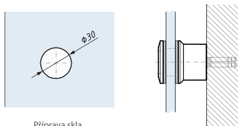
Příprava skla Glass preparation
