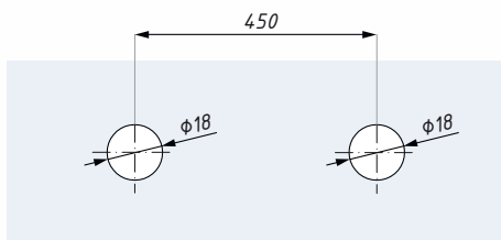
Příprava skla pro úchyt AJ51-TTG Glass preparation for clamb AJ51-TTG
