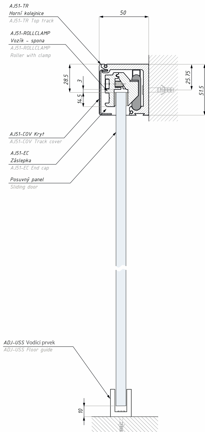
Montáž do stěny pro posuvné dveře Wall installation for sliding door
