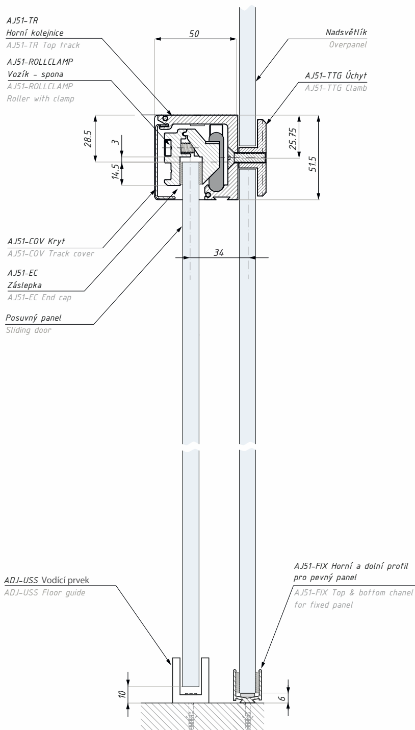
Montáž do pevného panelu Overpanel inocellation
