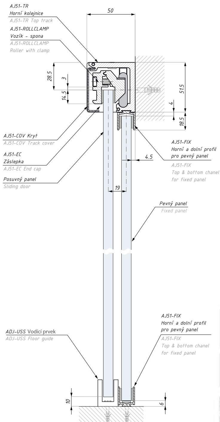
Montáž do stěny pro posuvné dveře s pevným panelem Wall installation for sliding door with fixed panel
