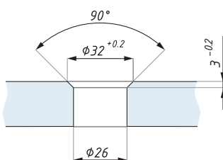
Příprava skla Glass preparation
