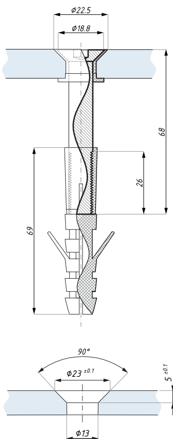
Příprava skla Glass preparation
