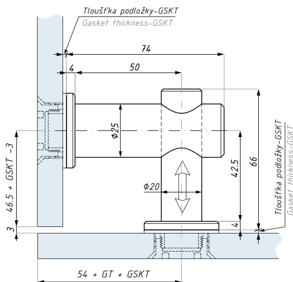
GT- Tloušťka skla / Glass thickness GSKT - Tloušťka podložky / Gasket thickness
