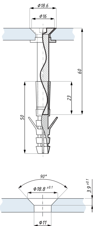
Příprava skla Glass preparation
