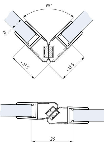
Těsnění PMFE 6-8 montáž na sklo 8 mm Clip seal PMFE 6-8 for glass 8 mm
