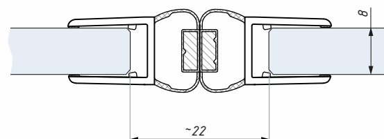
Těsnění PMBE 6-8 montáž na sklo 8mm Clip seal PMBE 6-8 for glass 8 mm
