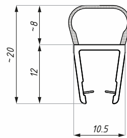
Těsnění ABE 6-8 Clip seal ABE 6-8
