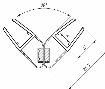
Těsnění PMFE 6-8 Clip seal PMFE 6-8
