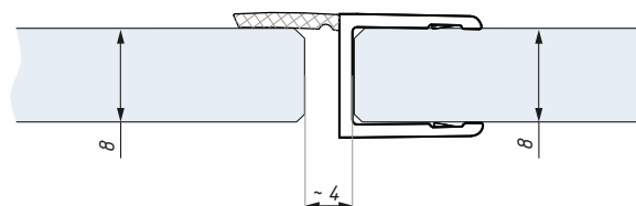
Těsnění WSE 6-8 montáž na sklo 8 mm Clip seal WSE 6-8 for glass 8 mm
