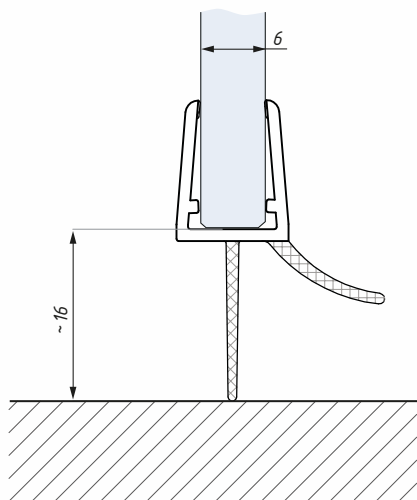
Těsnění BSE 6-8 montáž na sklo 6 mm Clip seal BSE 6-8 for glass 6 mm
