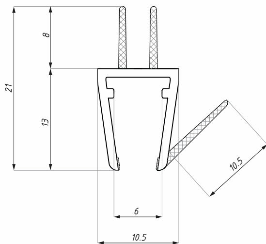
Těsnění WBE 6-8 Clip seal WBE 6-8
