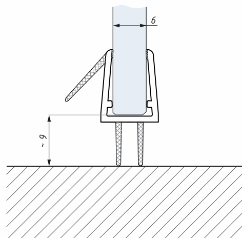
Těsnění WBE 6-8 montáž na sklo 6 mm Clip seal WBE 6-8 for glass 6 mm
