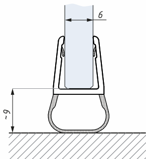
Těsnění ABE 6-8 montáž na sklo 6 mm Clip seal ABE 6-8 for glass 6 mm
