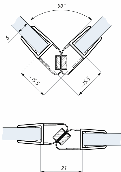
Těsnění PMFE 6-8 montáž na sklo 6 mm Clip seal PMFE 6-8 for glass 6 mm
