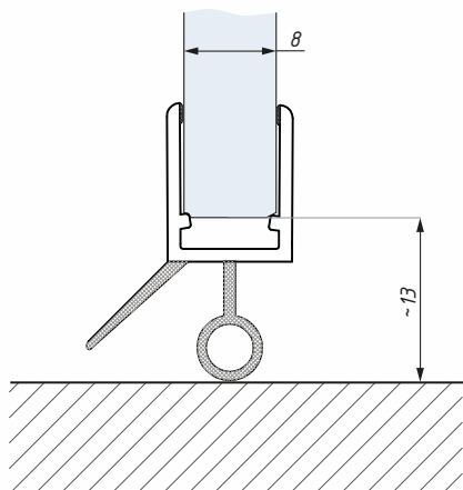
Těsnění DOE 6-8 montáž na sklo 8 mm Clip seal DOE 6-8 for glass 8 mm
