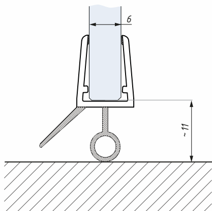
Těsnění DOE 6-8 montáž na sklo 6 mm Clip seal DOE 6-8 for glass 6 mm
