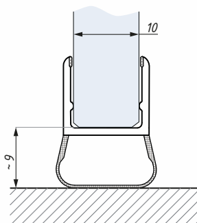
Těsnění ABE 10 montáž na sklo 10 mm Clip seal ABE10 for glass 10 mm
