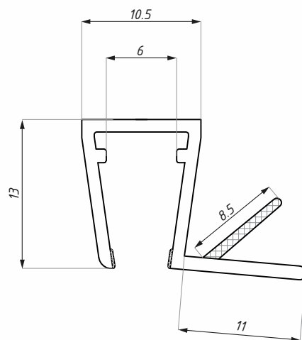
Těsnění ASE 6-8 Clip seal ASE 6-8
