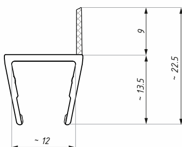
Těsnění WSE 8-10 Clip seal WSE 8-10
