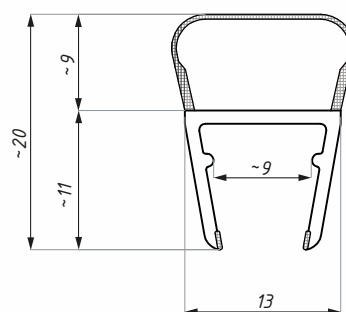
Těsnění ABE 10 Clip seal ABE 10
