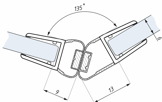
Těsnění PMSE 6-8 montáž na sklo 6 mm Clip seal PMSE 6-8 for glass 6 mm
