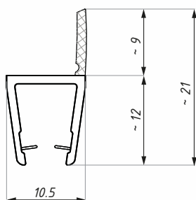
Těsnění WSE 6-8 Clip seal WSE 6-8
