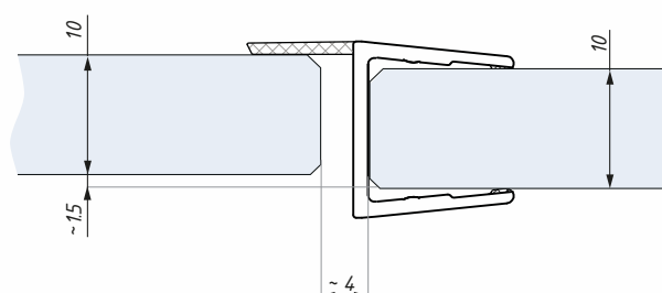
Těsnění WSE 8-10 montáž na sklo 10 mm Clip seal WSE 8-10 for glass 10 mm
