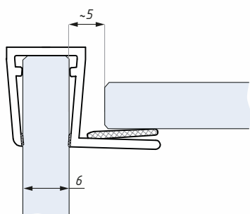
Těsnění ASE 6-8 montáž na sklo 6 mm Clip seal ASE 6-8 for glass 6 mm
