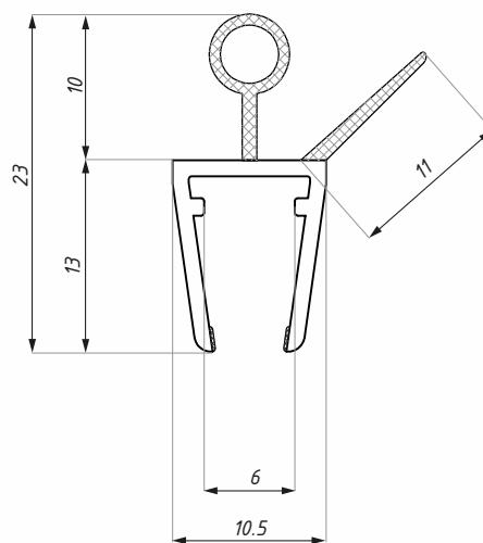
Těsnění DOE 6-8 Clip seal DOE 6-8
