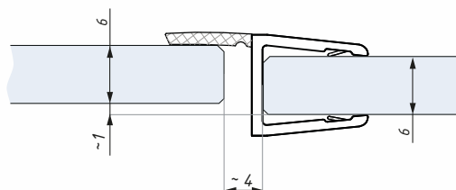
Těsnění WSE 6-8 montáž na sklo 6 mm Clip seal WSE 6-8 for glass 6 mm
