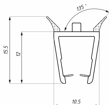
Těsnění GCE 6-8 Clip seal GCE 6-8
