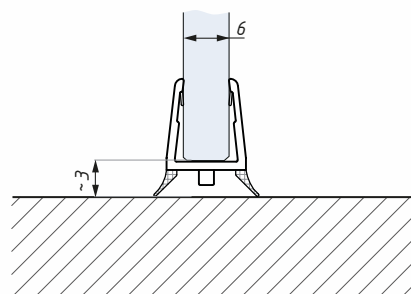
Těsnění GCE 6-8 montáž na sklo 6 mm Clip seal GCE 6-8 for glass 6 mm
