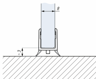
Těsnění GCE 6-8 montáž na sklo 8 mm Clip seal GCE 6-8 for glass 8 mm
