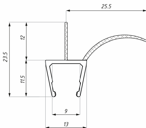
Těsnění GGE 8-10 Clip seal GGE 8-10
