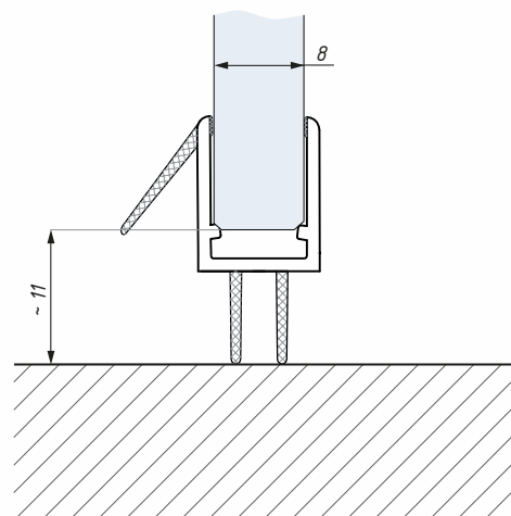
Těsnění WBE 6-8 montáž na sklo 8 mm Clip seal WBE 6-8 for glass 8 mm
