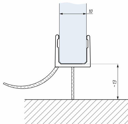
Těsnění GGE 8-10 montáž na sklo 10 mm Clip seal GGE 8-10 for glass 10 mm
