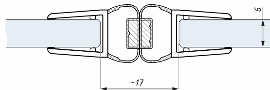
Těsnění PMBE 6-8 montáž na sklo 6 mm Clip seal PMBE 6-8 for glass 6 mm
