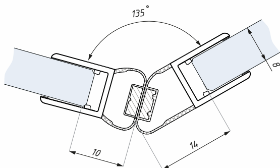
Těsnění PMSE 6-8 montáž na sklo 8 mm Clip seal PMSE 6-8 for glass 8 mm
