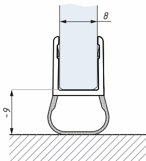
Těsnění ABE 6-8 montáž na sklo 8 mm Clip seal ABE 6-8 for glass 8 mm
