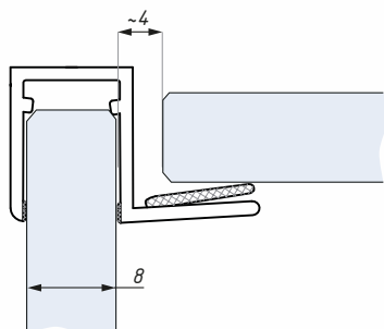
Těsnění ASE 6-8 montáž na sklo 8 mm Clip seal ASE 6-8 for glass 8 mm
