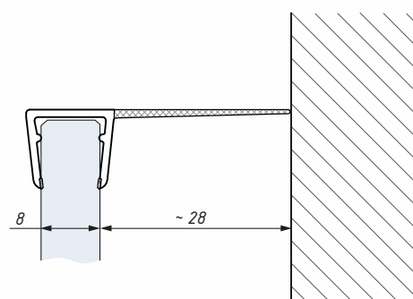
Těsnění SDE 8-10 montáž na sklo 8 mm Clip seal SDE 8-10 for glass 8 mm
