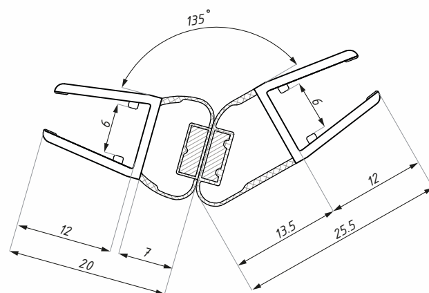
Těsnění PMSE 6-8 Clip seal PMSE 6-8
