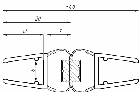
Těsnění PMBE 6-8 Clip seal PMBE 6-8
